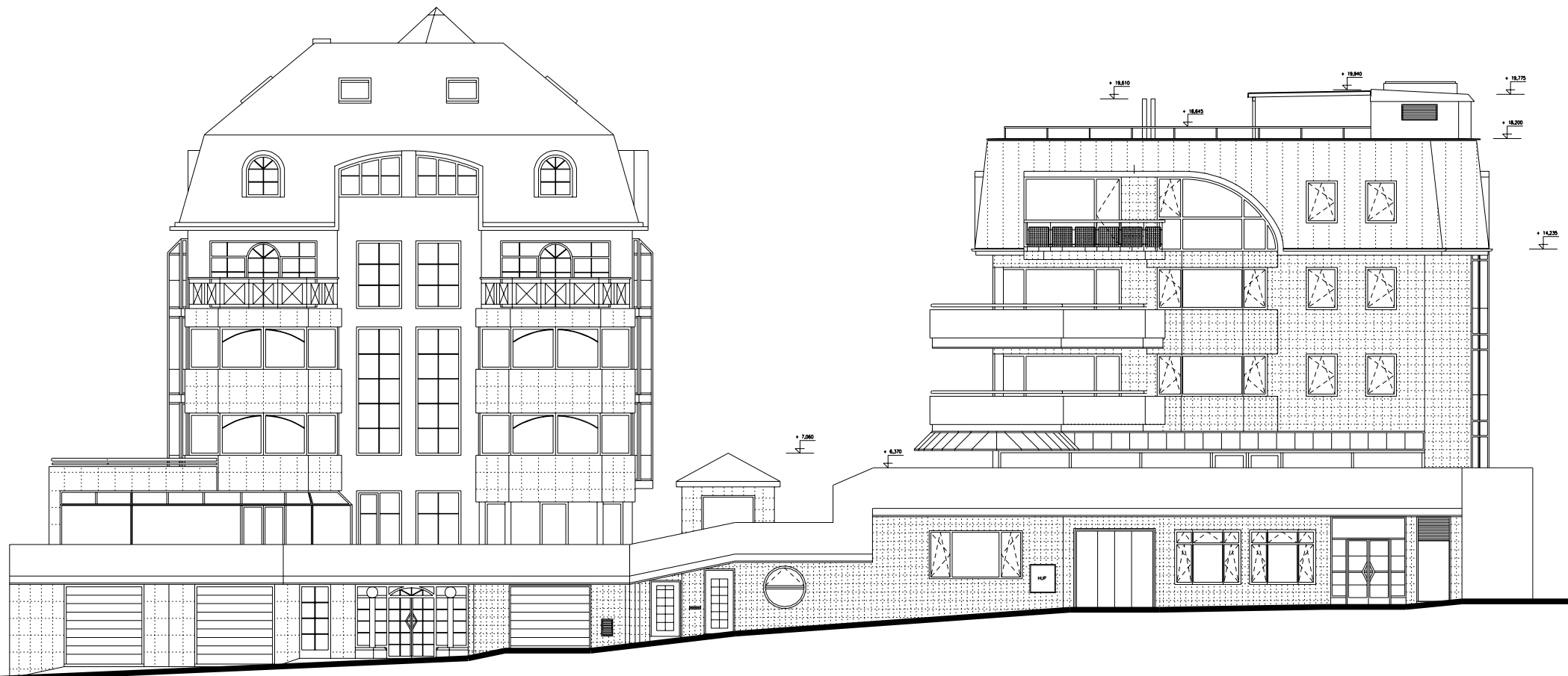
POHLED ZÁPADNÍ
